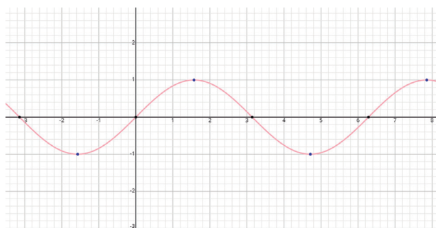
Figura 6. Gráfica de la función seno.
